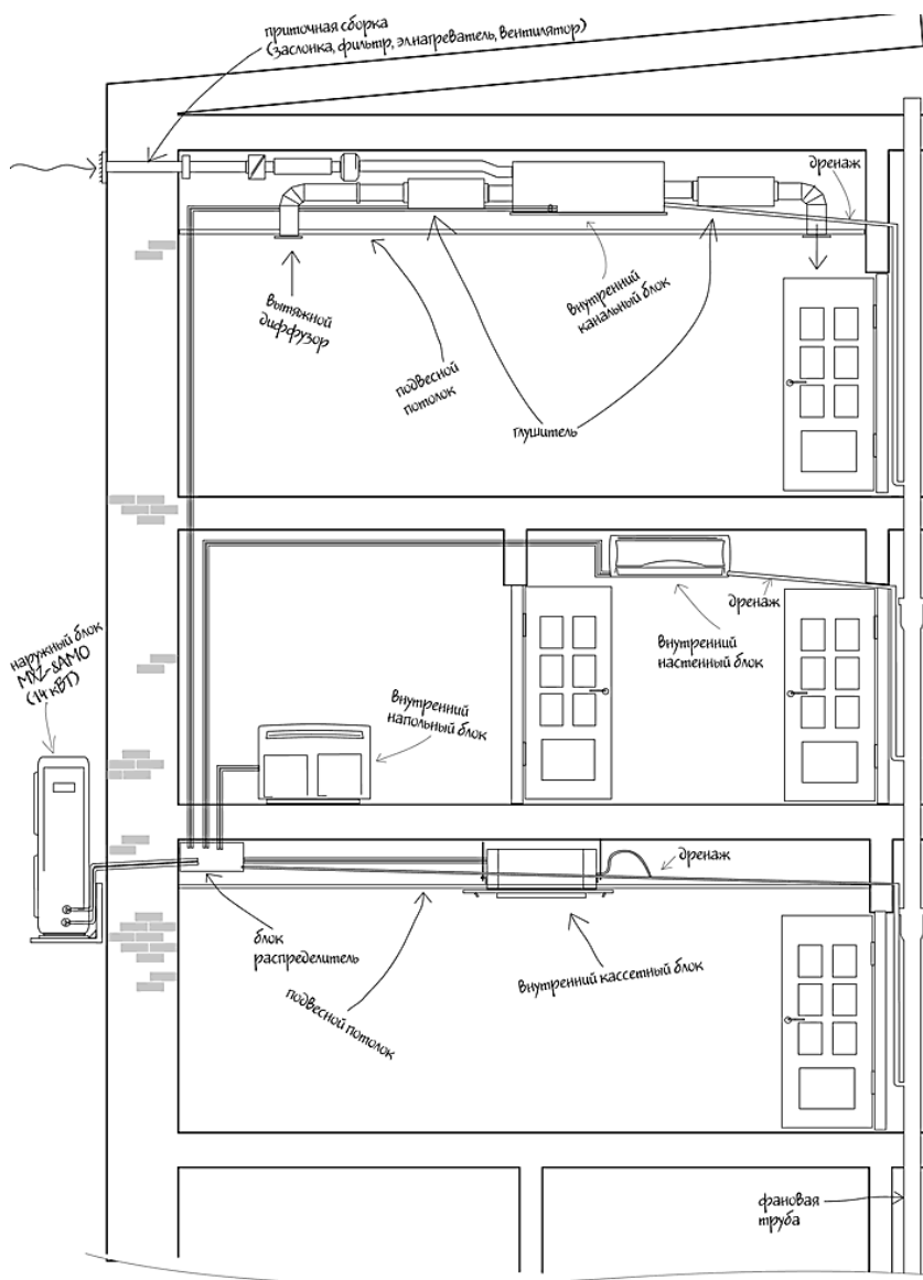
Рис. 3.15. Схема прокладки патрубков при кондиционировании нескольких помещений на разных этажах с помощью одного наружного и нескольких внутренних блоков
